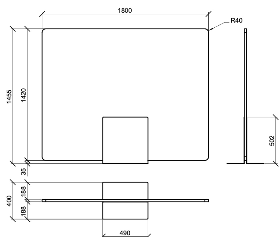
ECHOCOVE® STAND 180 L EC024STA180142A 1800 x 1455 x 400 mm
