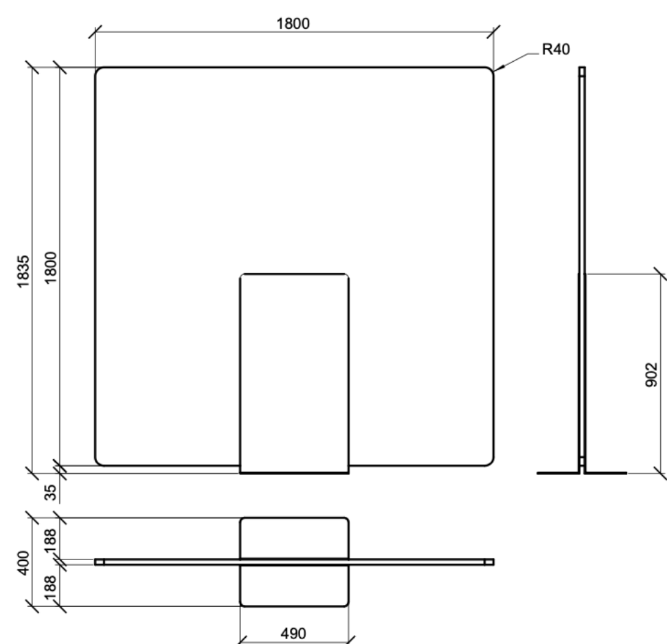
ECHOCOVE® STAND 180 XL EC024STA180180A 1800 x 1835 x 400 mm
