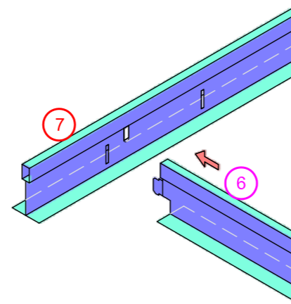
6 – Querprofil
