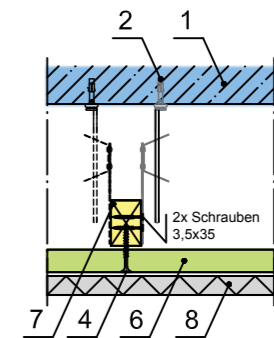
Längskantenstoß; Wechseln der Befestigungsstelle (Wechselnde Befestigung)
