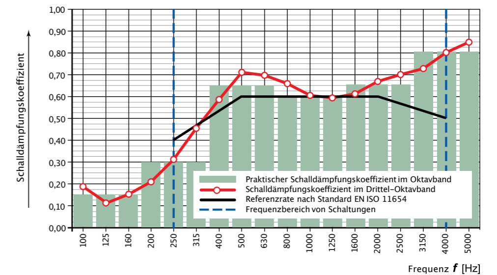
Praktischer Schalldämpfungskoeffizient nach Standard EN ISO 11654, \alpha_w : 0,60 Schalldämpfungs-kategorie nach EN ISO 11654:C
