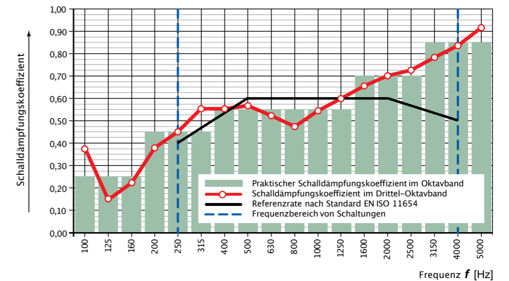
Praktischer Schalldämpfungskoeffizient nach Standard EN ISO 11654, \alpha_w : 0,60 Schalldämpfungsstufe nach EN ISO 11654: C
