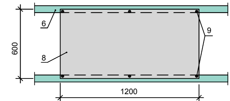
Befestigung von 600x1200 Platten mit 6 Schrauben in Längsrichtung
