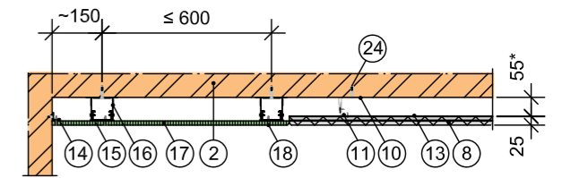
Horizontale Draufsicht der Eckenkonstruktion mit Gipskartonplatte
