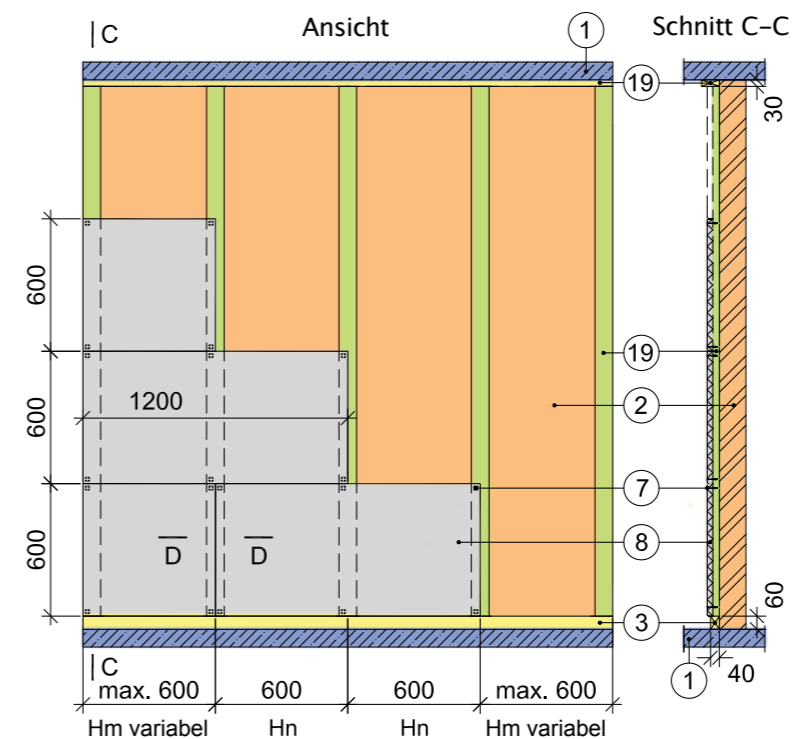
Befestigung von Holzlatten an der tragenden Wandkonstruktion
