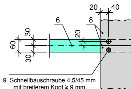
Befestigung von 600x1200 Platten mit 8 Schrauben
