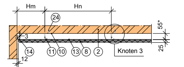
Horizontale Draufsicht der Eckenkonstruktion mit Schattenfuge
