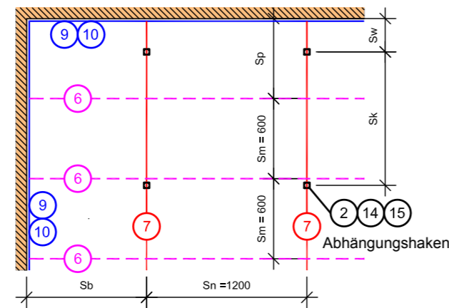
Profilanordnung für die Montage von 595x1195mm Platten d) S_n=1200 mm
