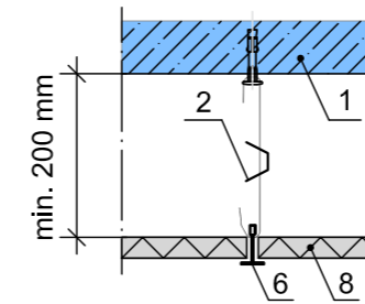
Montagehöhe – Schnellabhängung
