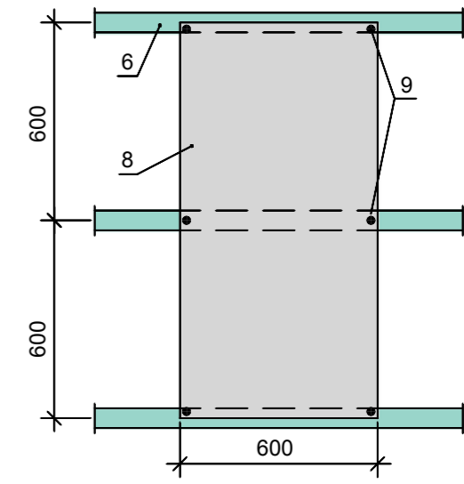
Befestigung von 600x1200 Platten mit 6 Schrauben
