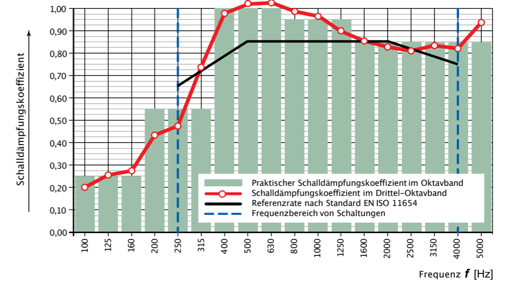
Praktischer Schalldämpfungskoeffizient nach Standard EN ISO 11654, \alpha_w : 0,85 Schalldämpfungs-klasse nach EN ISO 11654: B
