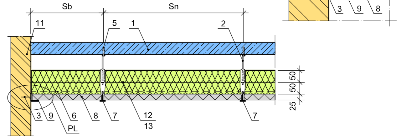
Abschnitt B1-B1, Profilanordnung für 595x595mm Platten
