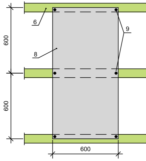
Befestigung von 600x1200 Platten mit 6 Schrauben
