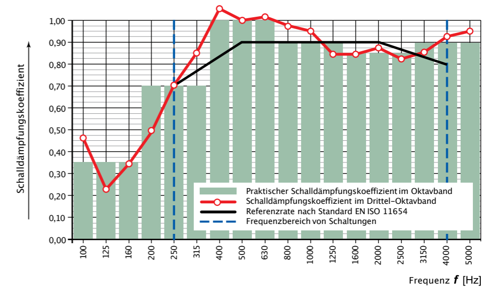
Praktischer Schalldämpfungskoeffizient nach Standard EN ISO 11654, \alpha_w : 0,90 Schalldämpfungs-kategorie nach EN ISO 11654:A
