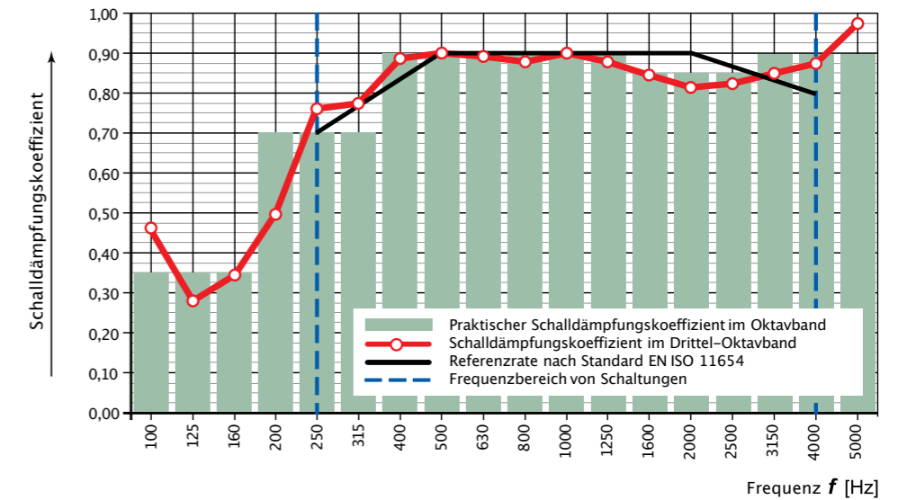
Praktischer Schalldämpfungskoeffizient nach Standard EN ISO 11654, \alpha_w : 0,90 Schalldämpfungsstufe nach EN ISO 11654: A
