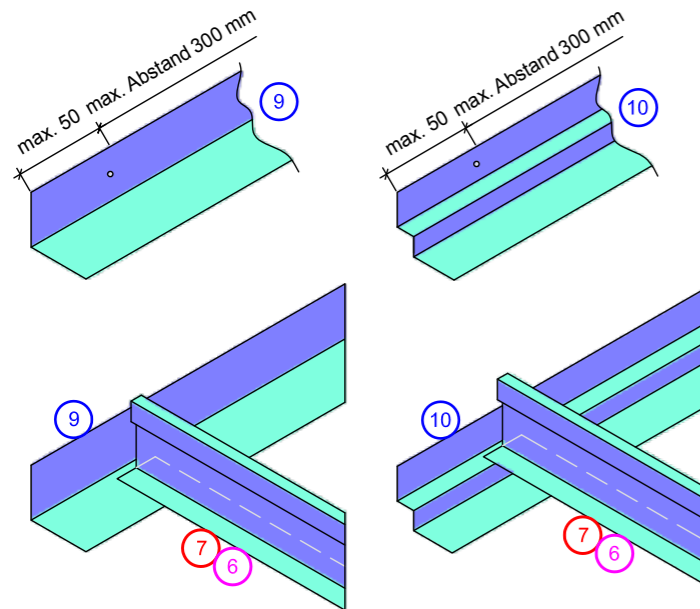
9; 10 – Umlaufende Profile, Montage
