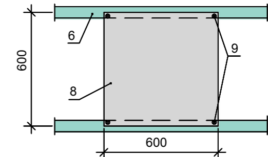
Befestigung von 600x600 Platten mit 4 Schrauben
