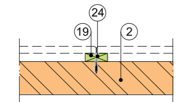
Befestigung von Holzlatten an der tragenden Wandkonstruktion
