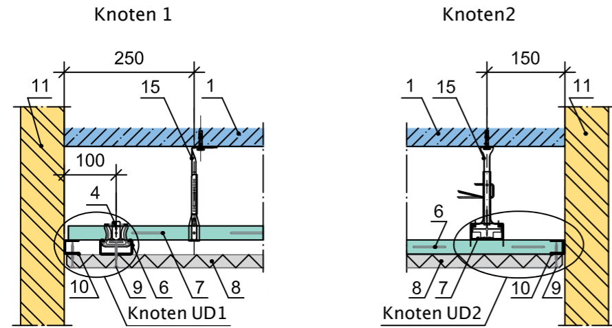
Stirnkantenstoß Anschluss an Wand
