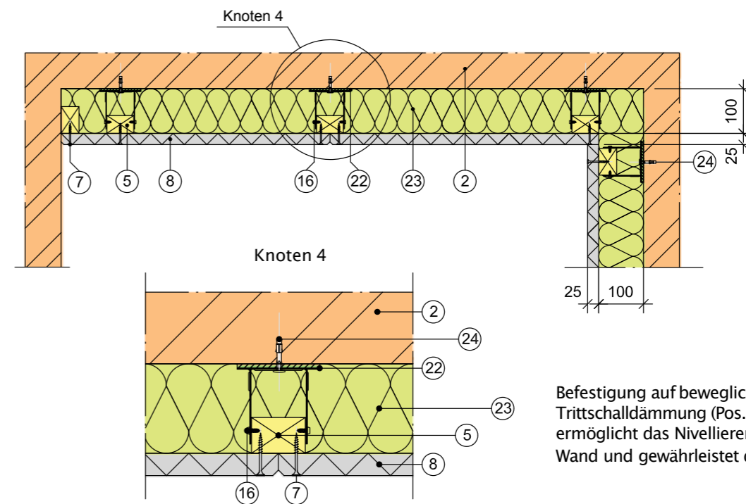
Befestigung auf beweglichem Untergrund
