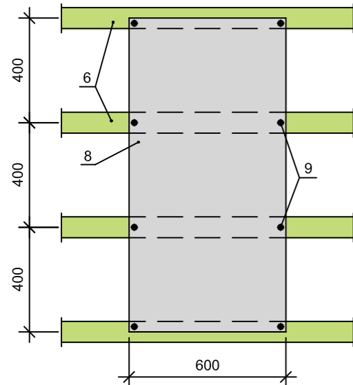
Befestigung von 600x1200 Platten mit 8 Schrauben
