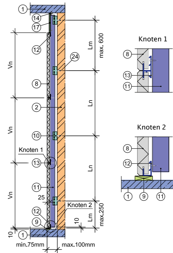
Vertikale Seitenansicht der Wand
