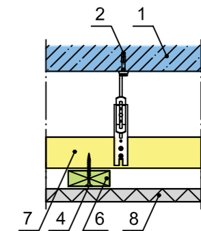
Stirnkantenstoß, Traglatte 40x60 mm
