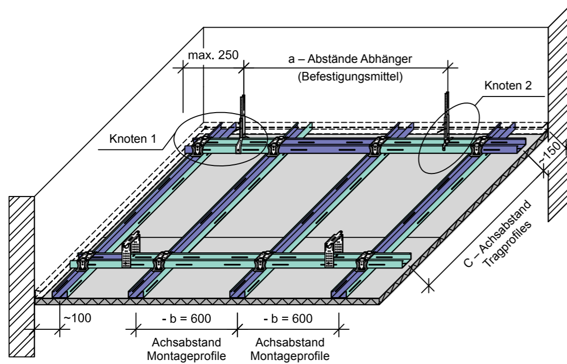
Montageabstand für Profile -600 mm
