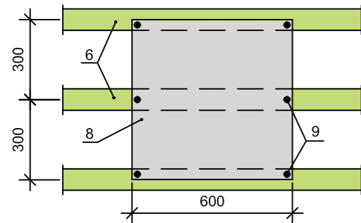
Befestigung von 600x600 Platten mit 6 Schrauben
