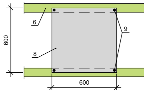
Befestigung von 600x600 Platten mit 4 Schrauben
