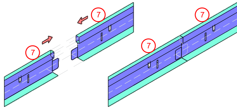
9; 10 – Umlaufende Profile, Montage
