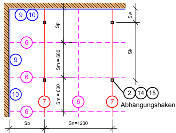
Profilanordnung für die Montage von 595x595mm Platten b) S_n=1200 mm
