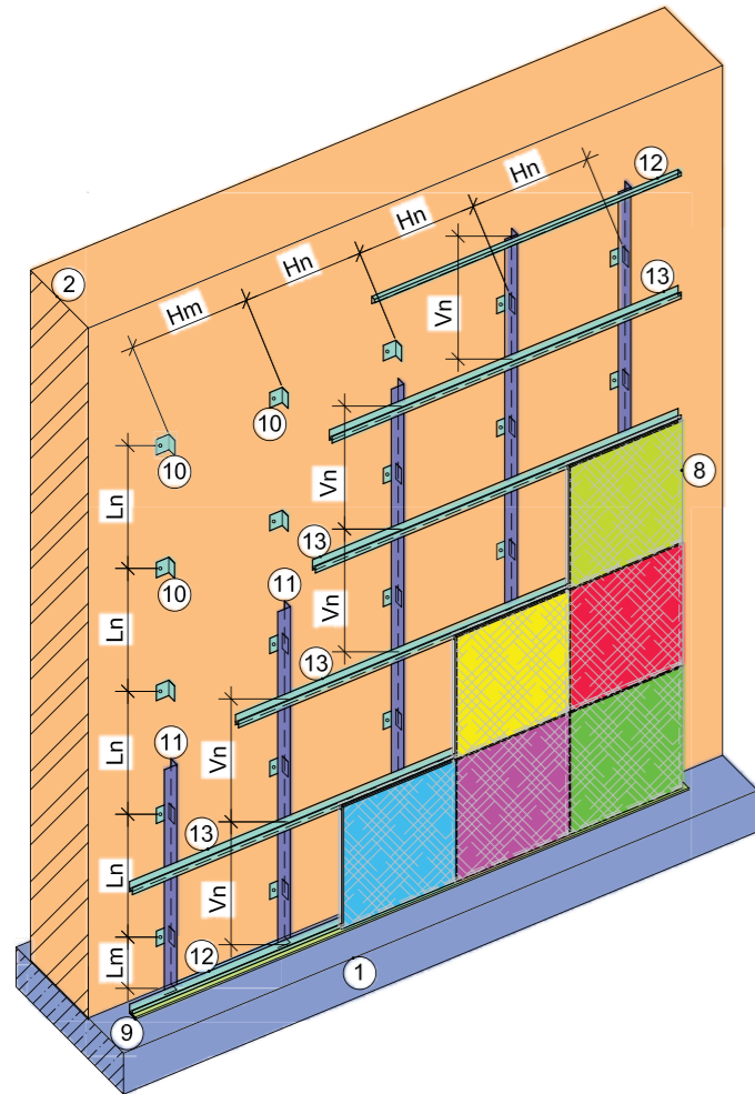
Montageschema der Befestigungsprofile
