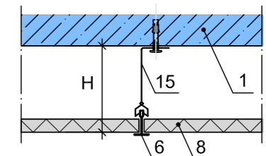
Montagehöhe – höhenverstellbarer Haken
