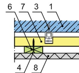
Stirnkantenstoß, Direktabhängiger 0,40 kN.
