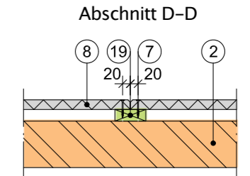
Befestigung von Holzlatten an der tragenden Wandkonstruktion
